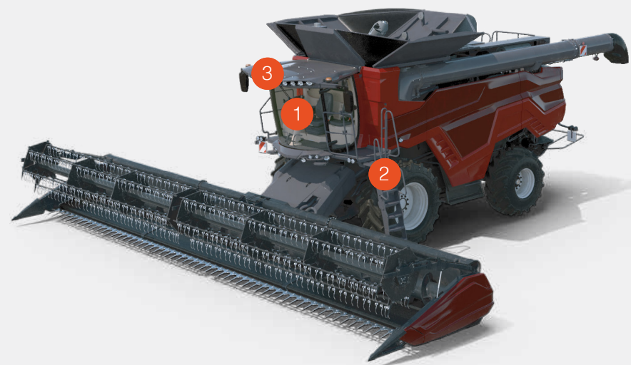
Przód
